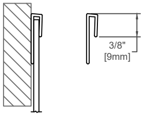
TOP CAP
