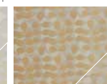
Spin
